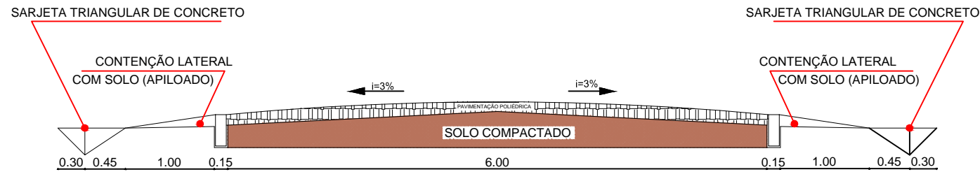
01 PERFIL TRANSVERSAL
