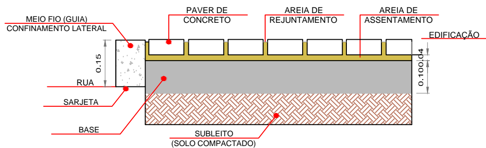
04 DETALHES PAVER
