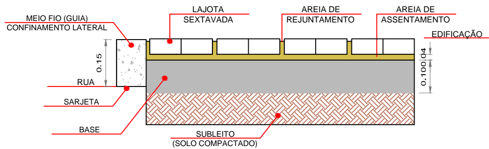
03 DETALHES LAJOTA
