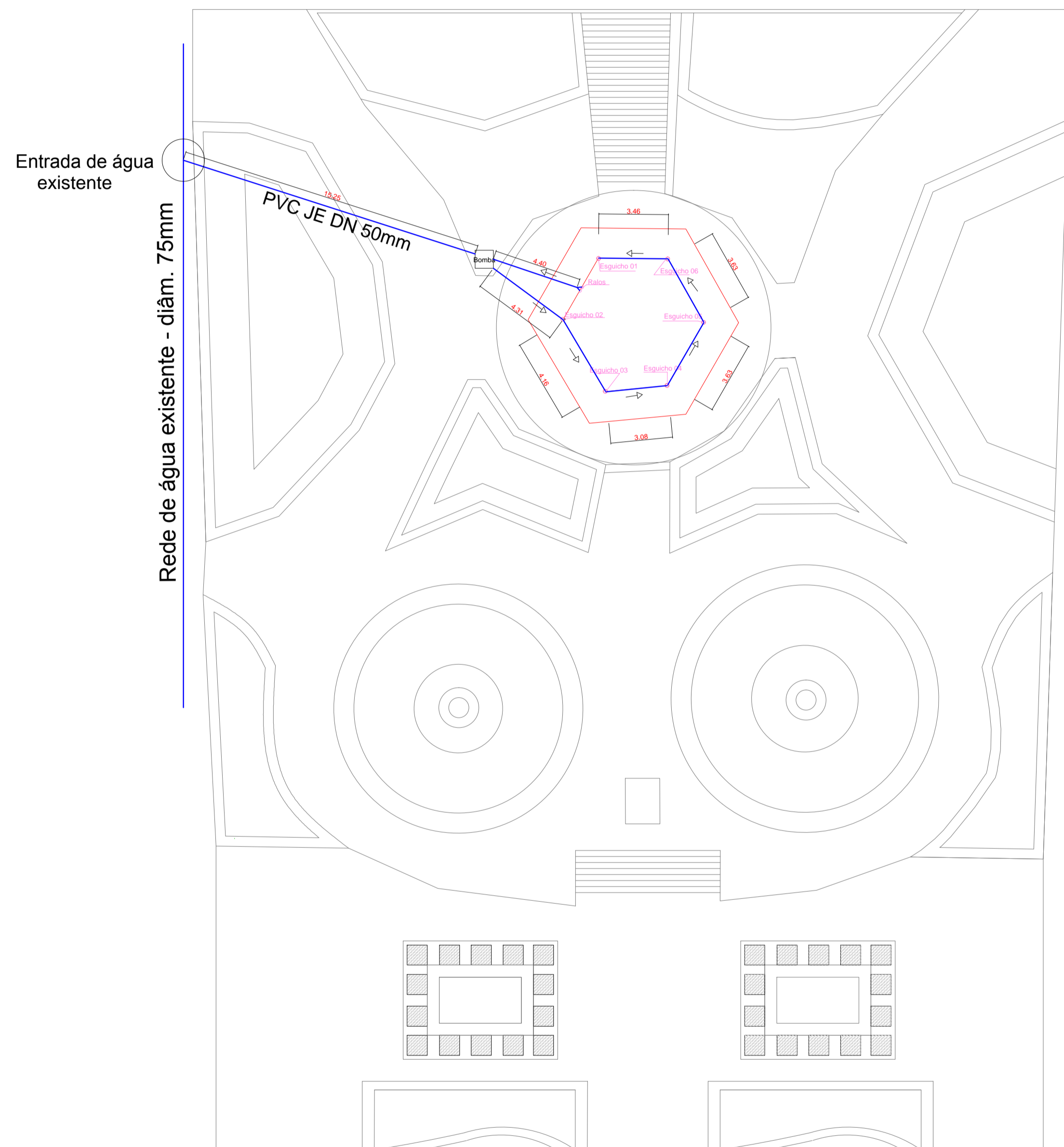
PLANTA BAIXA ESCALA 1:250
