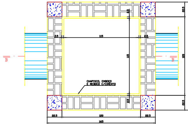
CORTE AA
