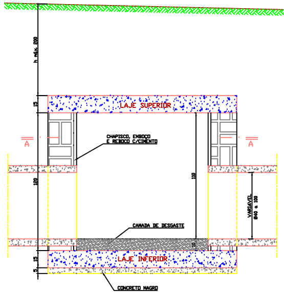
CORTE BB
