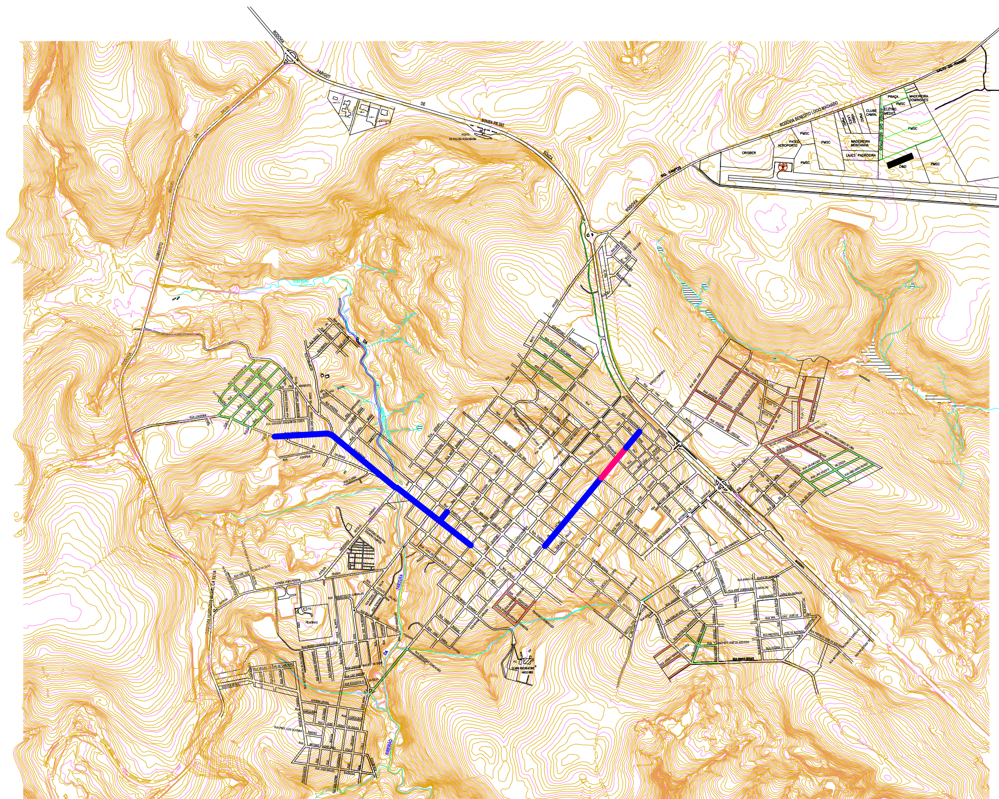
PLANTA DE LOCALIZAÇÃO DA INTERVENÇÃO
