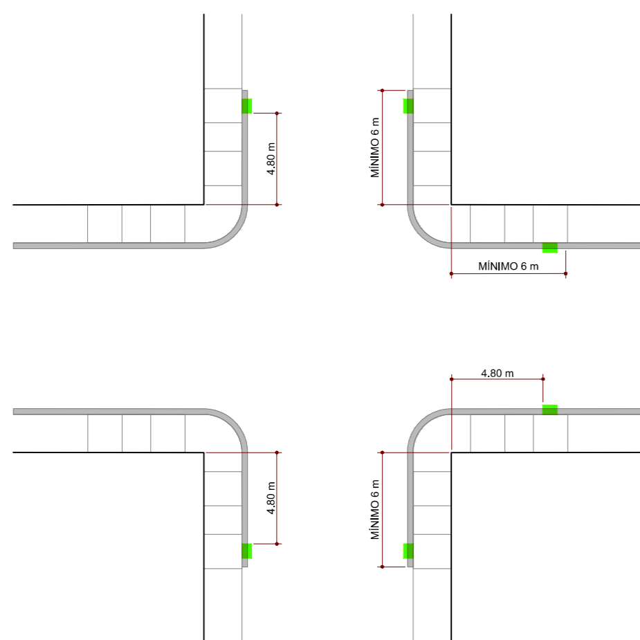
3 DETALHE 03 - LOCAÇÃO DAS BOCAS DE LOBO SEM ESCALA
