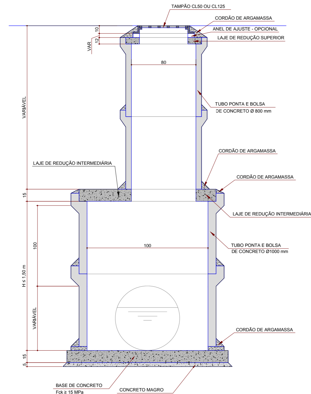
2 DETALHE 02 - POÇO DE VISITA SEM ESCALA
