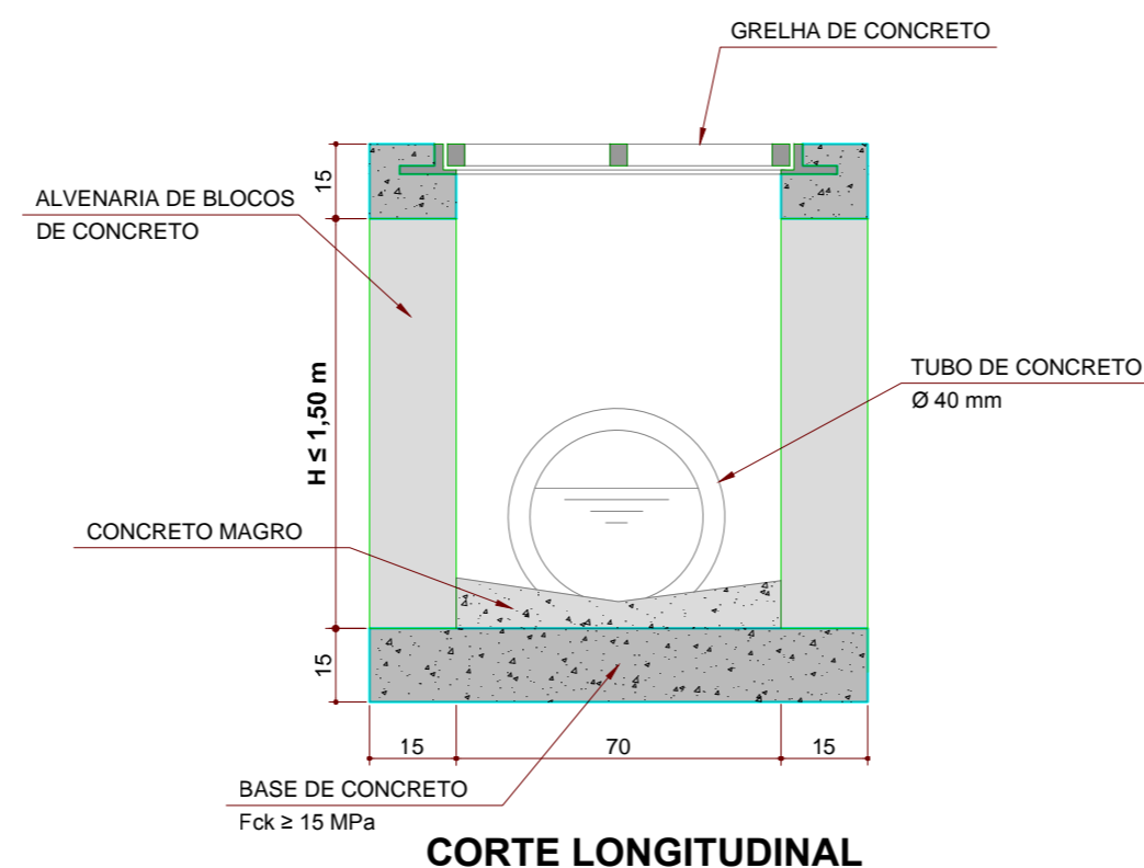
CORTE LONGITUDINAL
