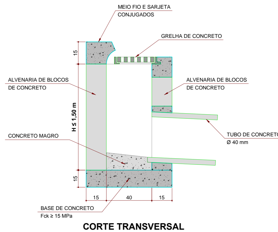
1 DETALHE 01 - BOCA DE LOBO SEM ESCALA
