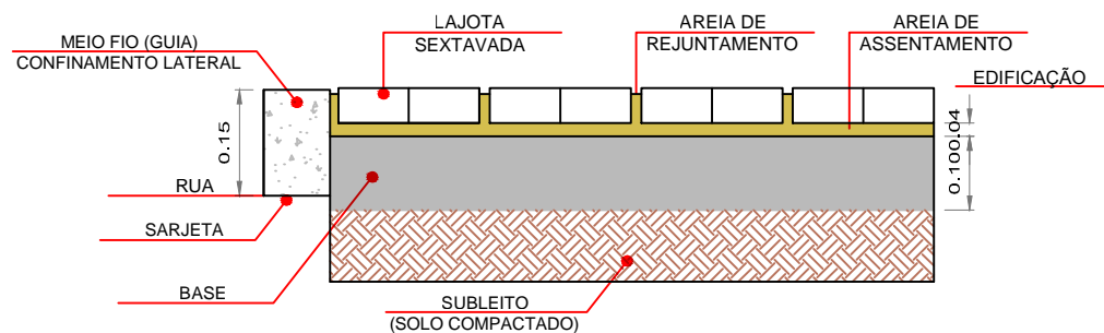
03 DETALHES LAJOTA
