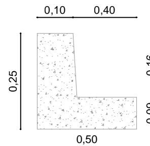
05 MEIO FIO COM SARJETA
