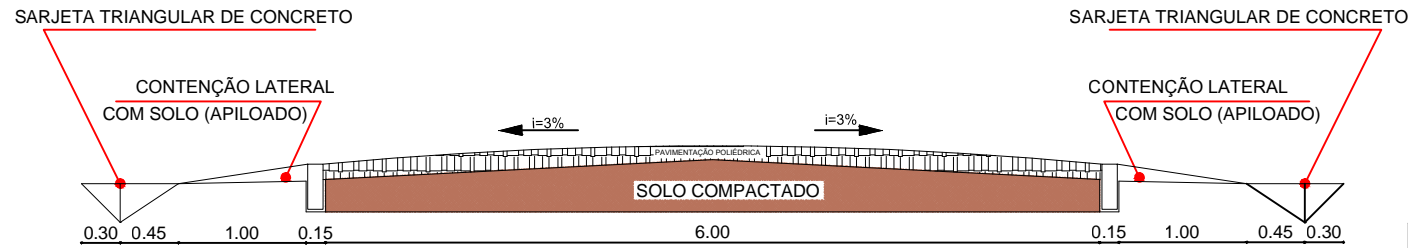
01 PERFIL TRANSVERSAL
