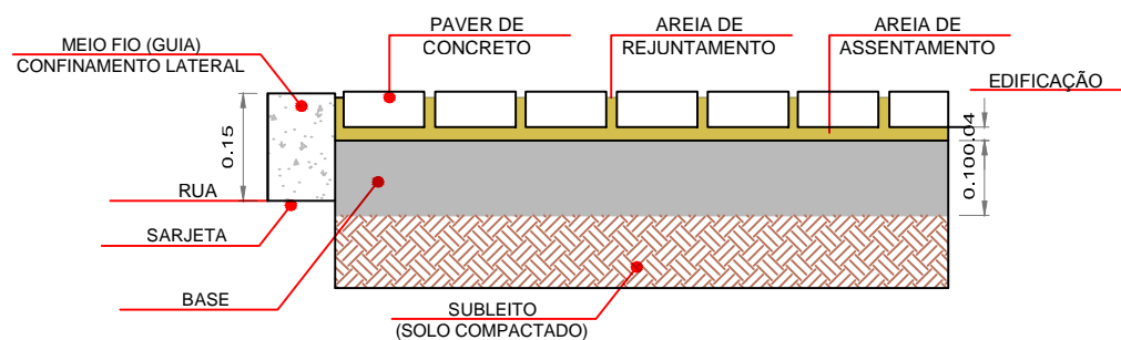
04 DETALHES PAVER
